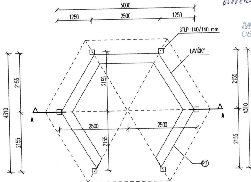
PODORYS M 1:100
