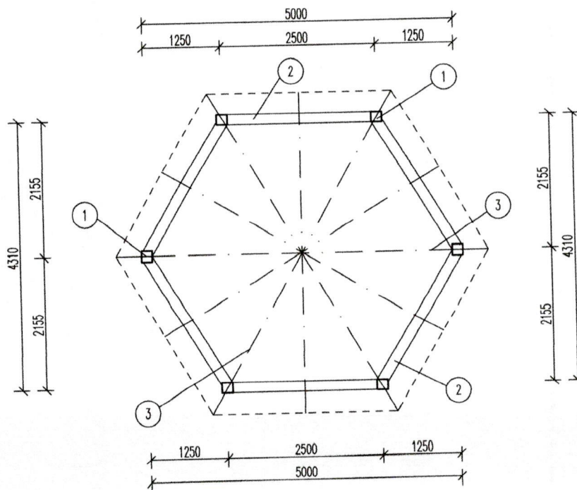
PÔDORYS KROVU M 1:100
